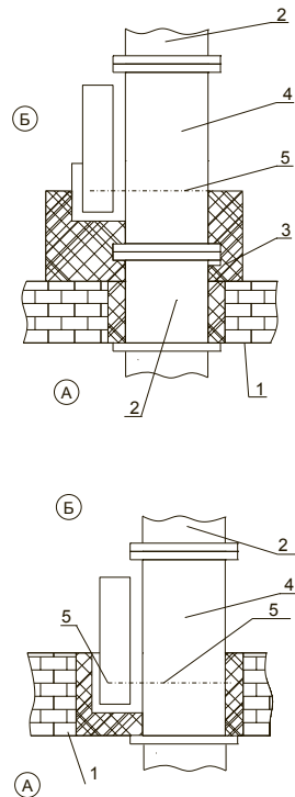
Схема установки клапана КСП-2
